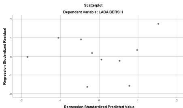
Gambar 1. Uji Heteroskedastisitas
