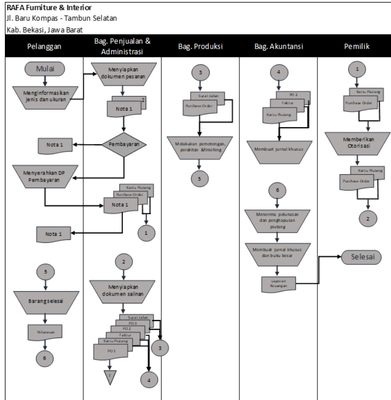
Gambar 9. Rancangan Flowchart
